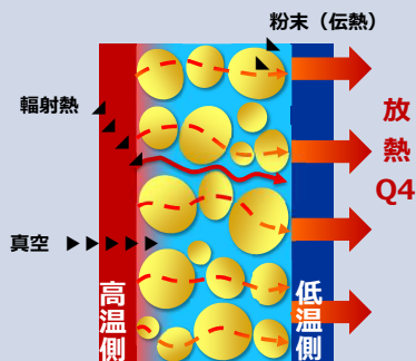
図-4 粉末真空断熱
