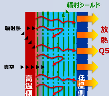
図-5 積層真空断熱
