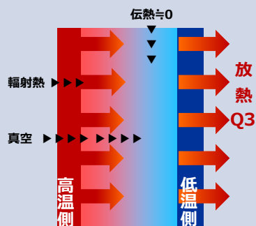
図-3 真空断熱
